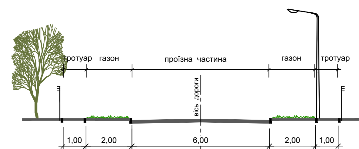
Поперечні профілі вулиць М 1:100
